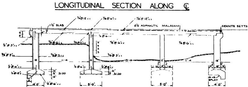
Fig. 342.—Longitudinal Section.
